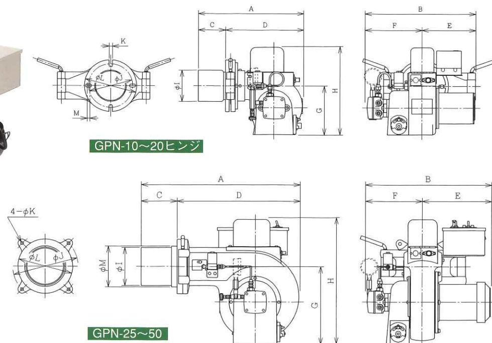
ヒンジタイプ
