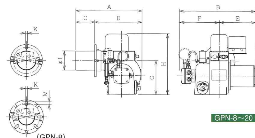
フランジ固定タイプ
